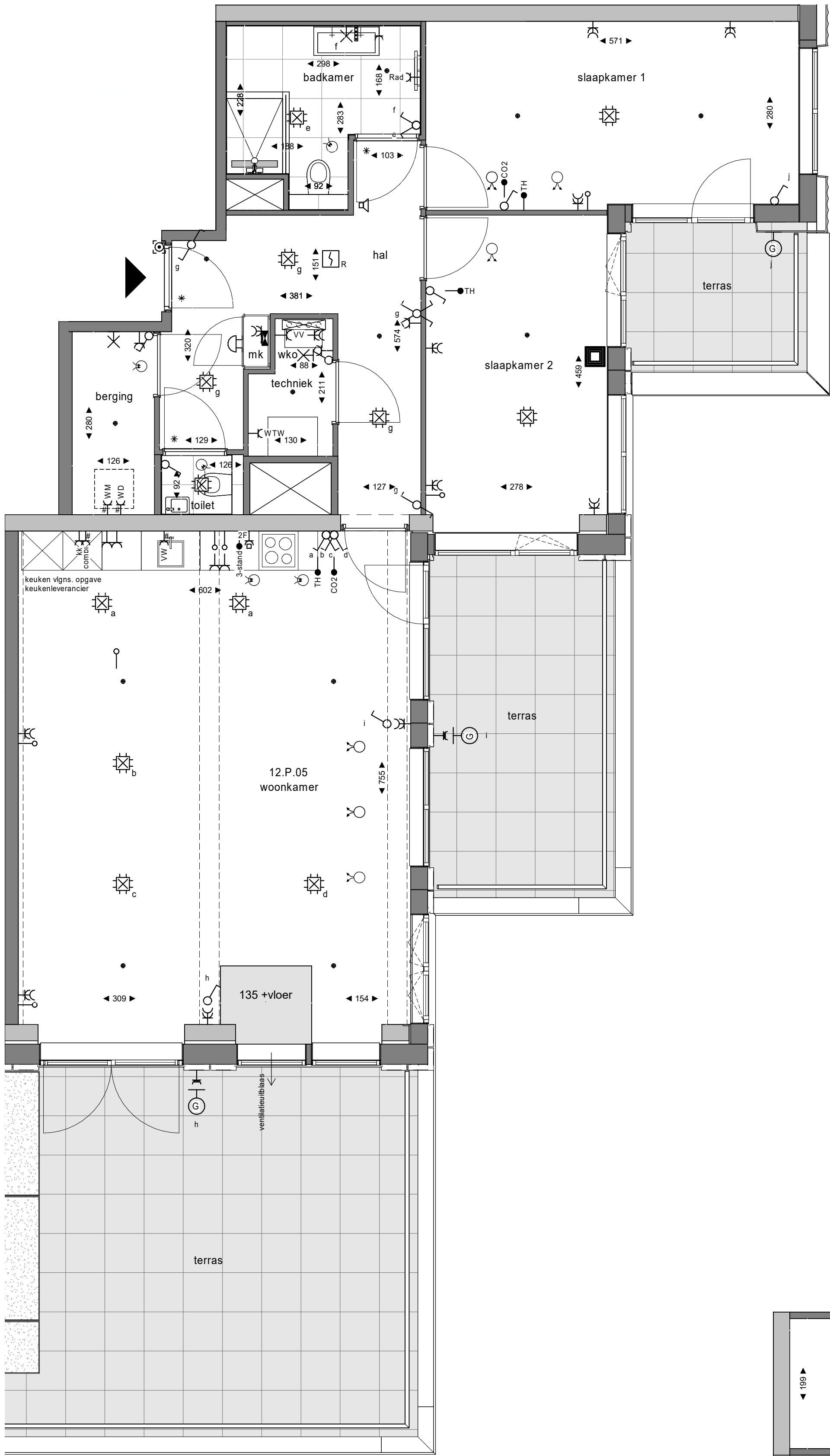
plattegrond 1 : 50 12e verdieping
